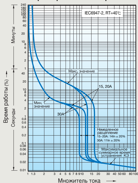
Характеристические кривые
