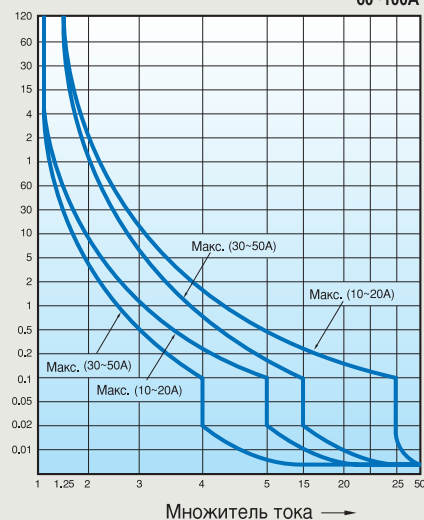
Характеристические кривые 60-100A
