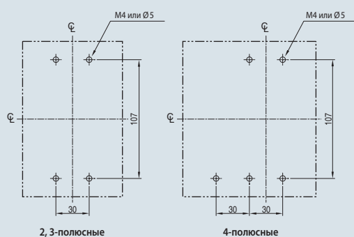
Разметка отверстий
