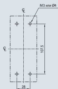
Разметка отверстий
