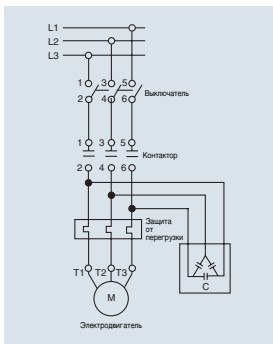
Емкостная цепь
