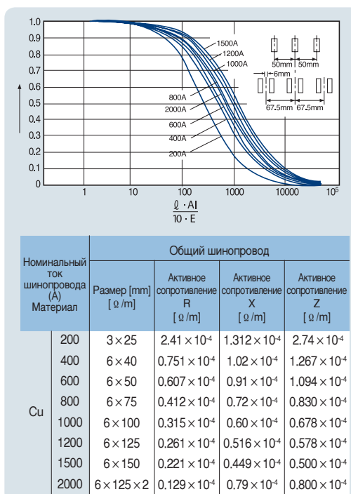
Рис. 10. Понижающий коэффициент для общей шины (медной)
